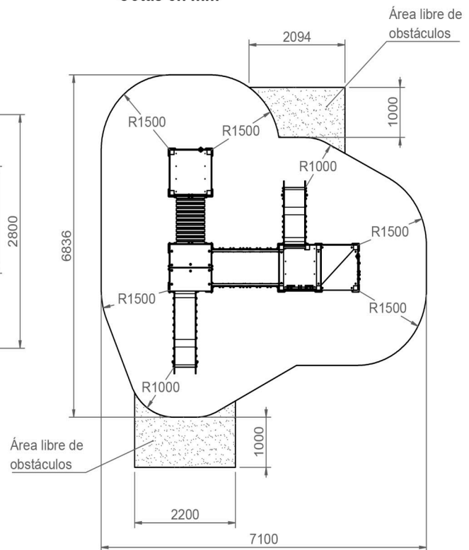
PLANTA Área de Seguridad 36.5m 2 Cotas en mm
