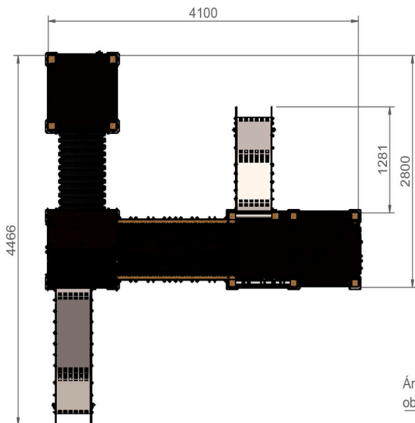
PLANTA Cotas en mm
