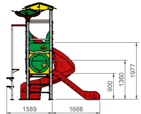
PERFIL IZQ Cotas en mm
