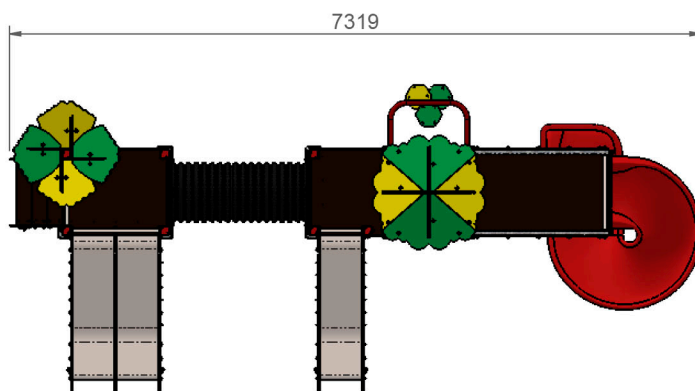
PLANTA Cotas en mm
