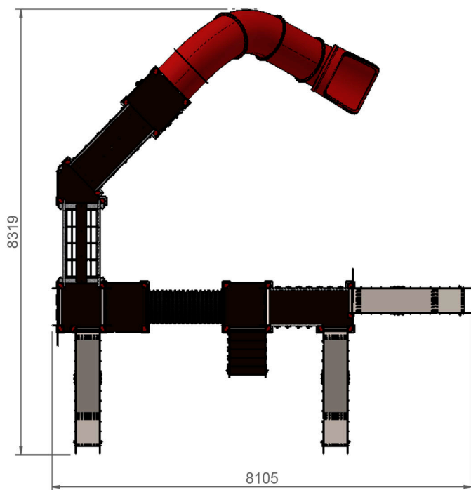
PLANTA Cotas en mm
