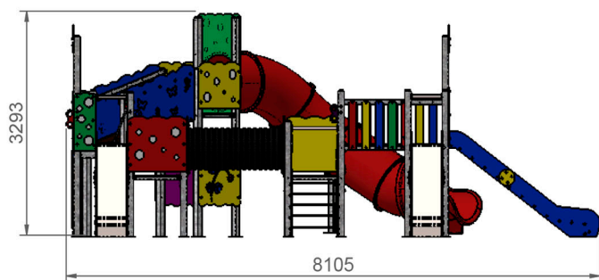
ALZADO Cotas en mm
