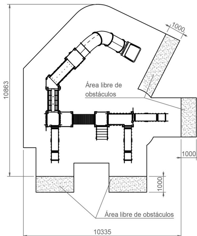
PLANTA Área Seguridad = 82m 2 Cotas en mm
