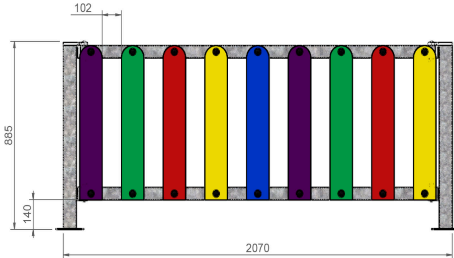
ALZADO Cotas en mm
