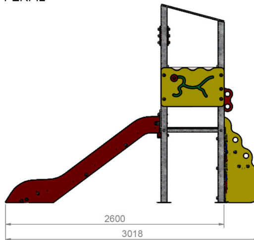
PERFIL
