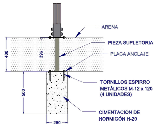
DETALLE DE CIMENTACIÓN EN ARENA
