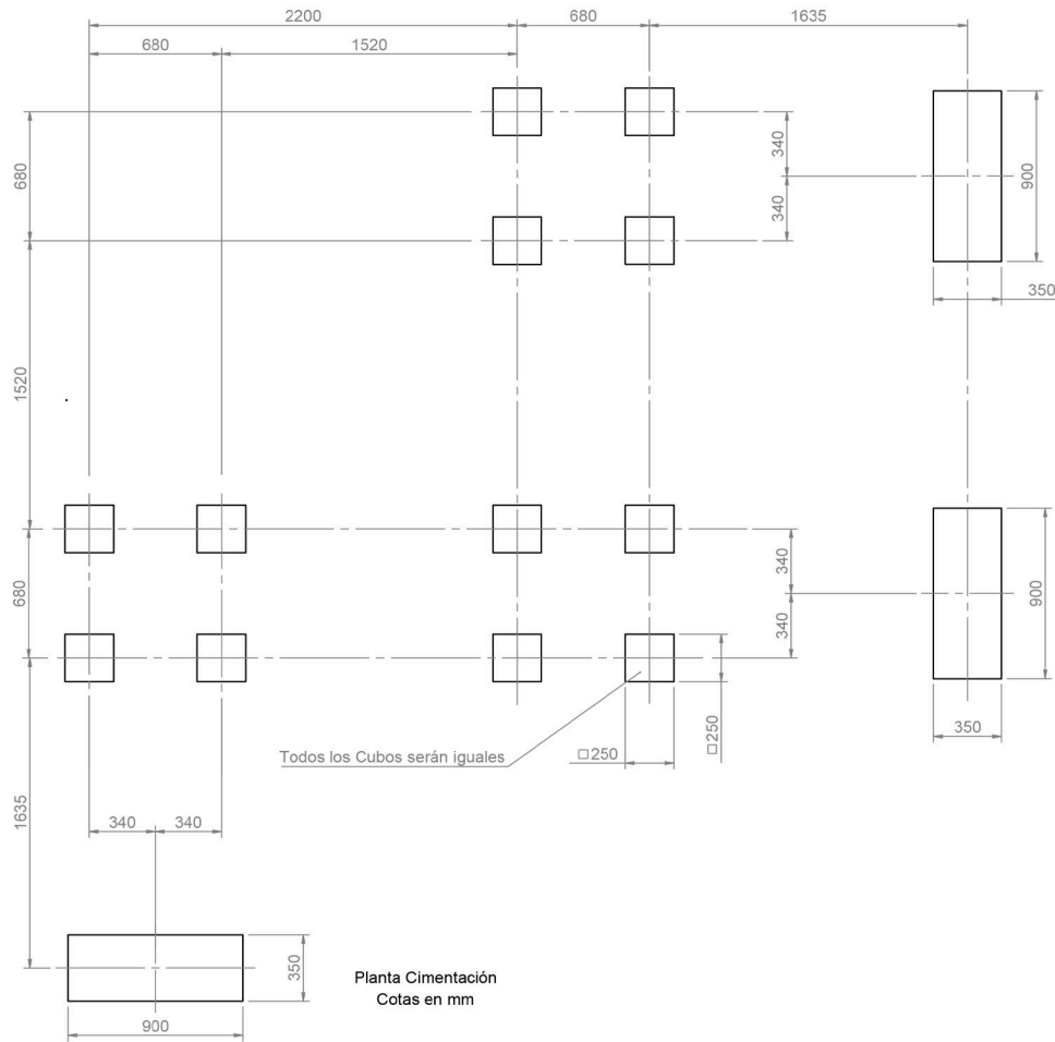
DETALLE DE CIMENTACIÓN EN ARENA
