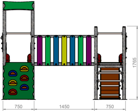
ALZADO
