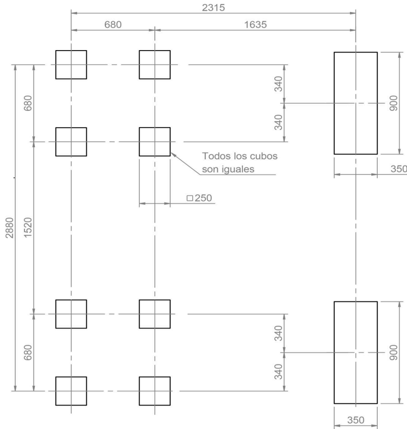
Planta Cimentación Cotas en mm
