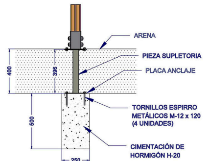
DETALLE DE CIMENTACIÓN EN ARENA
