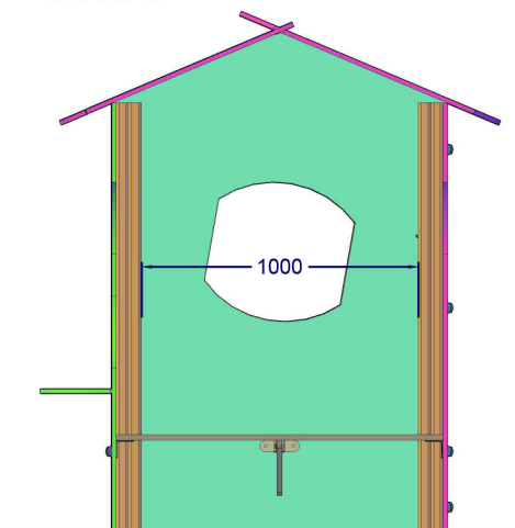
Sección
